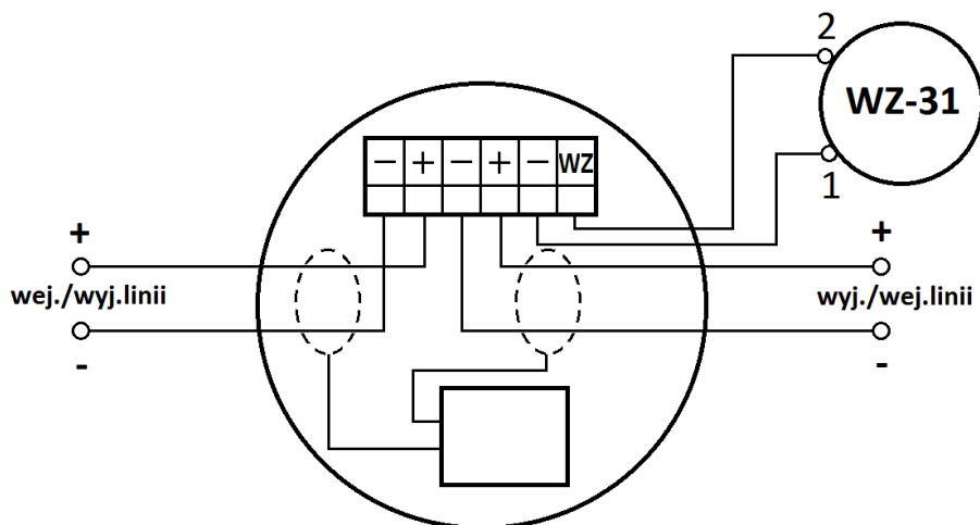
Rys.7.1 Schemat połączeń stosowany dla czujki pracującej w zerowym trybie dodatkowym.
