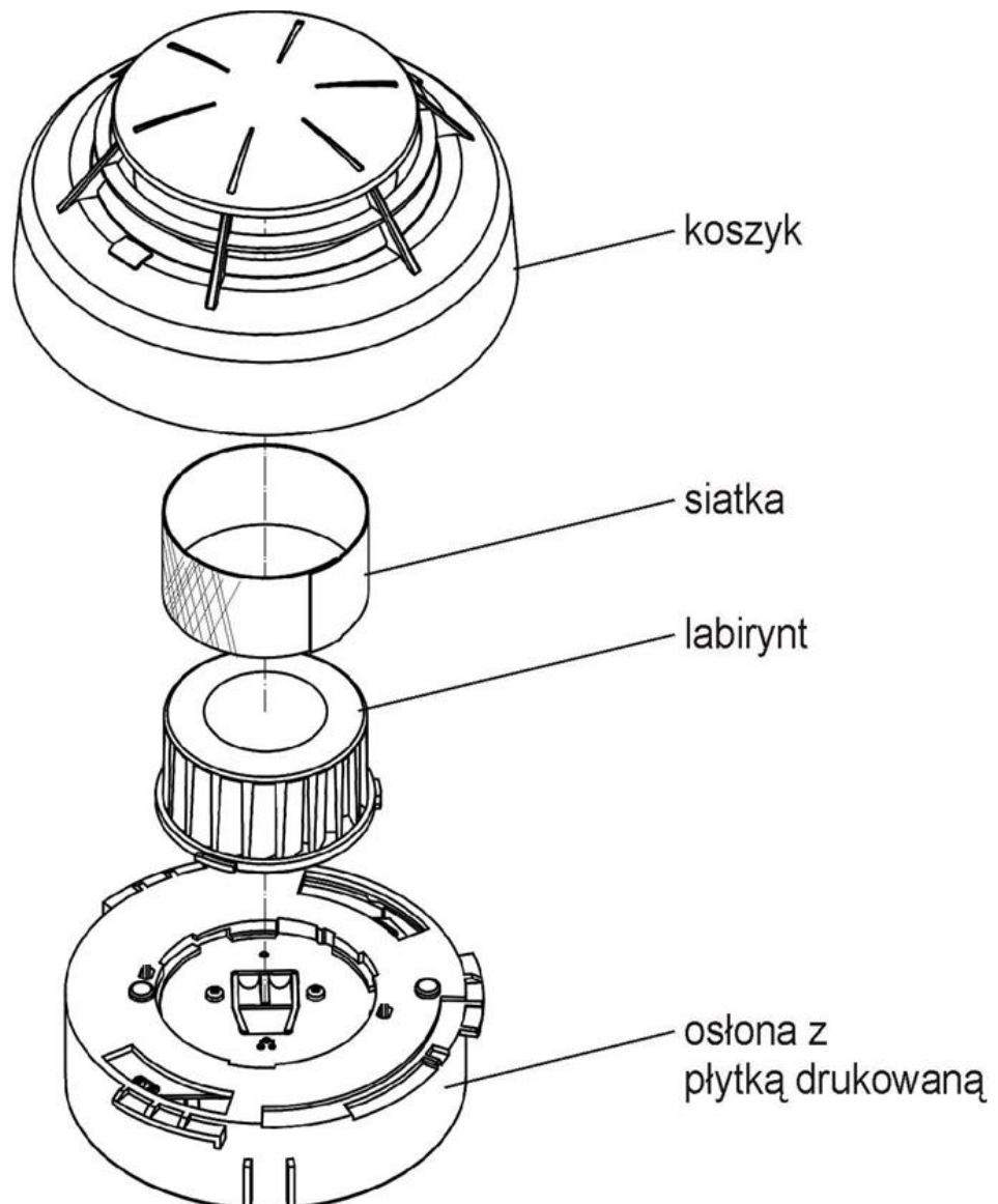
Rys.5.2 Elementy czujki po demontażu
